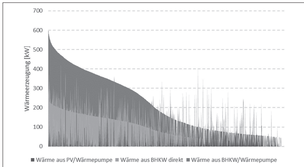
Abbildung 7: Erzeugungsverlauf Pth-Szenario 2
