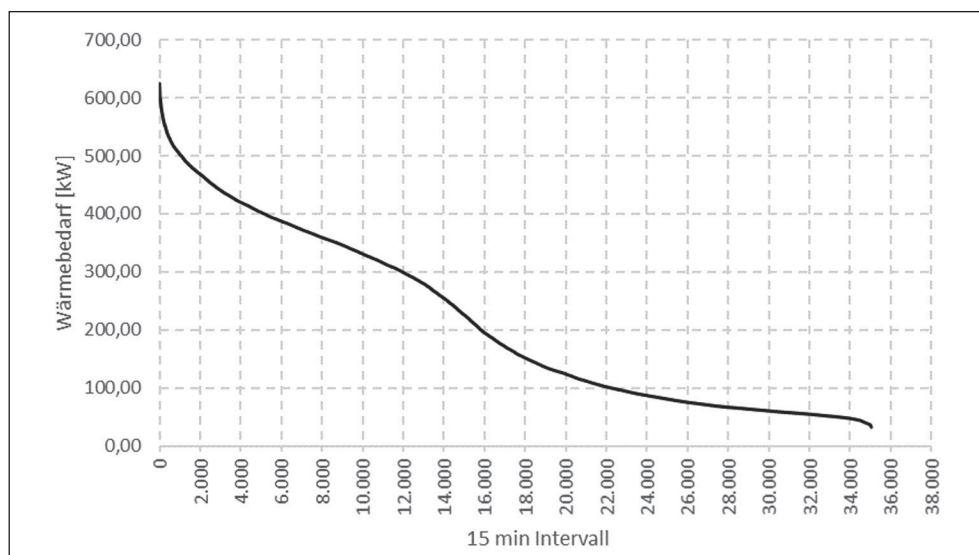
Abbildung 3: Jahresdauerlinie Wärmelast
