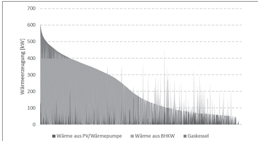
Abbildung 5: Erzeugungsverlauf Pth-Szenario 1
