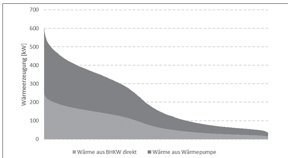
Abbildung 6: Erzeugungsverlauf Pth-Szenario 2
