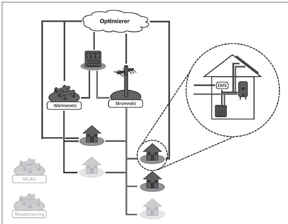
Abbildung 1: Hybrid Grids Demo-Ansatz
