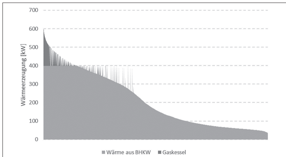
Abbildung 4: Erzeugungsverlauf Referenzszenario
