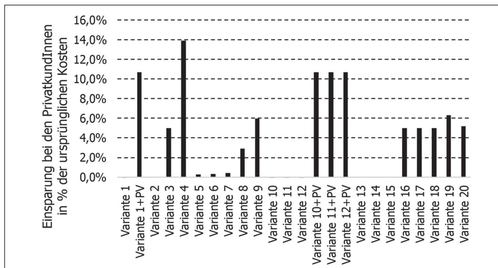
Abbildung 2: Einsparungen bei den EndkundInnen durch die Nutzung der Flexibilität
