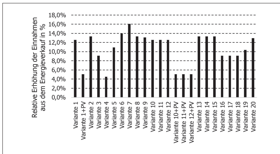
Abbildung 8: Relative Steigerung der Einnahmen des Energieversorgers durch den Flexibilitätseinsatz
